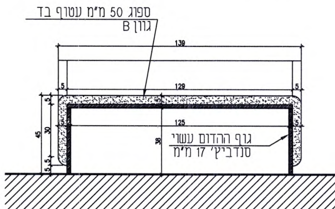
חתך A-A
