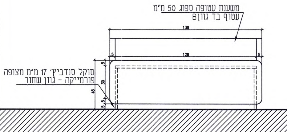
מבט 01
