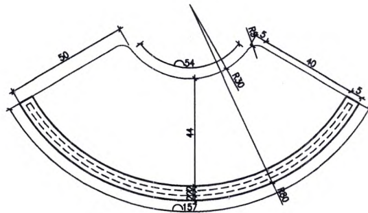
מבט על
