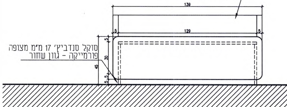
מבט 01
